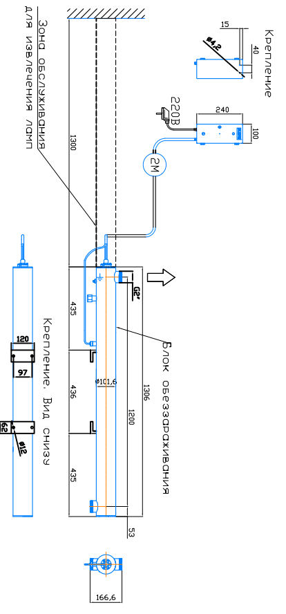
При установке протока выходной патрубок увеличивается на 97,5 мм Масштаб 1:1, редакция 02.02.2022 год
