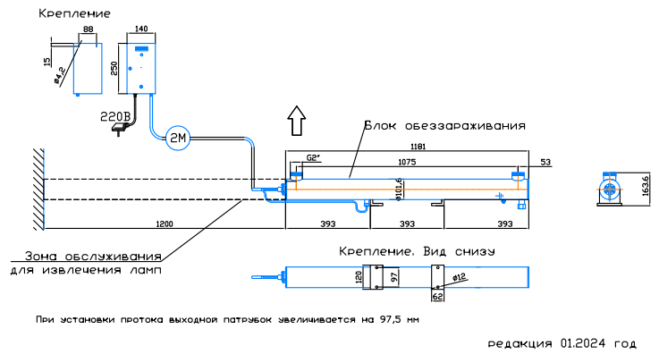
Монтажный чертёж установки ОДВ-15 (ОДВ-6С). Патрубки - П. Изготовление под заказ. Горизонтальное расположение
