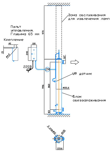
Монтажный чертёж установки ОДВ-5 (ОДВ-2С) Патрубки - П. Изготовление под заказ Вертикальное расположение
