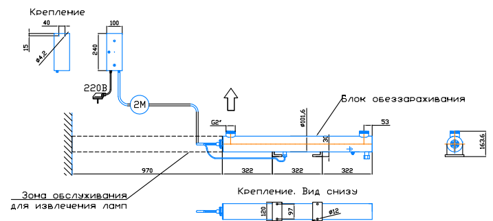
Монтажный чертёж установки ОДВ-5 (ОДВ-2С). Патрубки - П. Изготовление под заказ. Горизонтальное расположение
