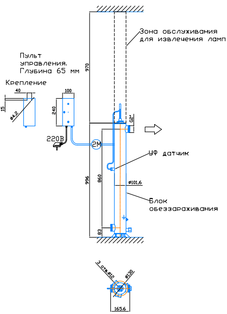
Монтажный чертёж установки ОДВ-5 (ОДВ-2С) Патрубки - И. Стандартное изготовление Вертикальное расположение
