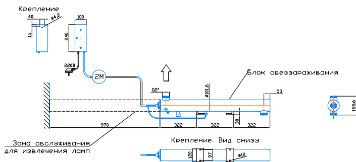
Монтажный чертёж установки ОДВ-5 (ОДВ-2С). Патрубки - И. Изготовление под заказ. Горизонтальное расположение
