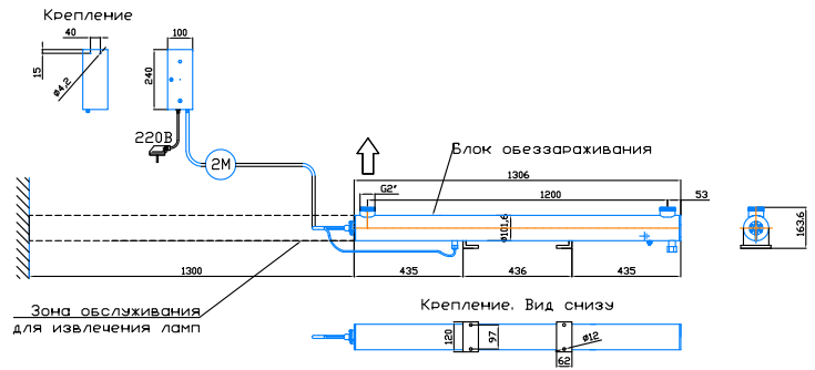
При установке протока выходной патрубков увеличивается на 97,5 мм Масштаб 1:1, редакция 12.2022 год
