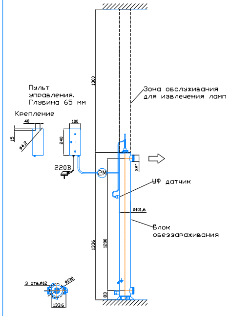
При установке протока выходной патрубков увеличивается на 97,5 мм Масштаб 1:1, редакция 12.2022 год
