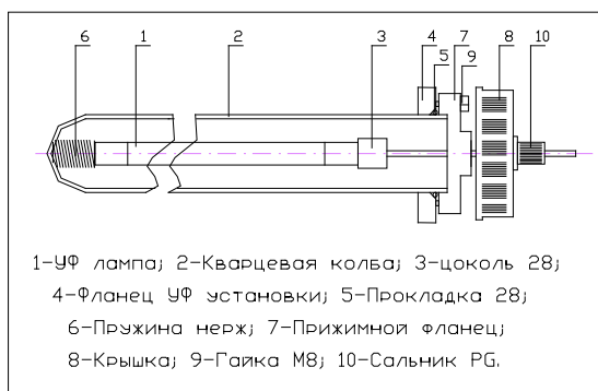
Рис. 2 Узел сборки лампы
