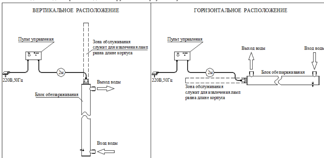
Рис. 1 Общий вид установки типа «ОДВ» расположение установки
