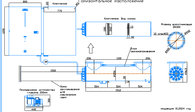
Монтажный чертёж установки ОДВ-300СА (ОДВ-700А). Патрубки - П. Изготовление под заказ. Горизонтальное расположение
