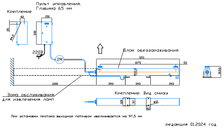
Монтажный чертёж установки ОДВ-20 (ОДВ-8С). Патрубки - П. Изготовление под заказ. Горизонтальное расположение
